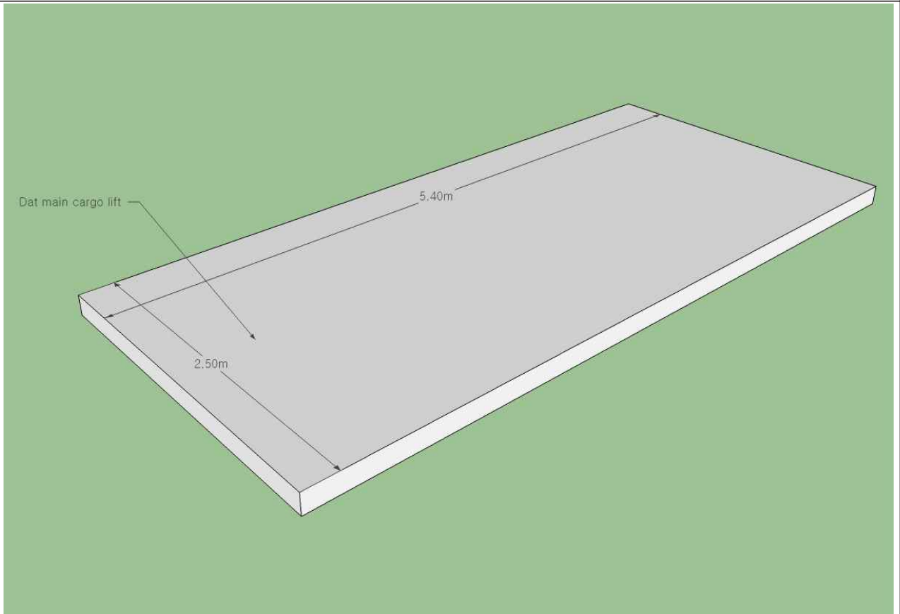
무대반입 리프트
